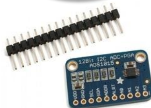
ADS1015 Module
