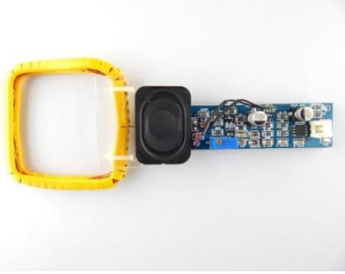
Metal Detector
